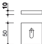
..... VEILIGHEIDSRUZET VIERKANT MET KERN TREKBEVELIGING
